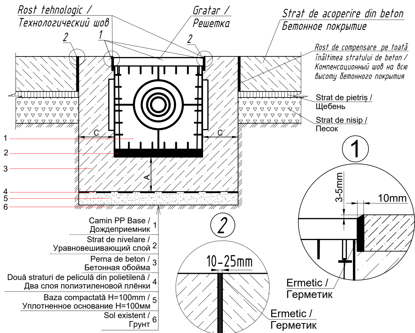
Parametrii recomandati pentru perna de beton / Рекомендуемые параметры бетонной обоймы
